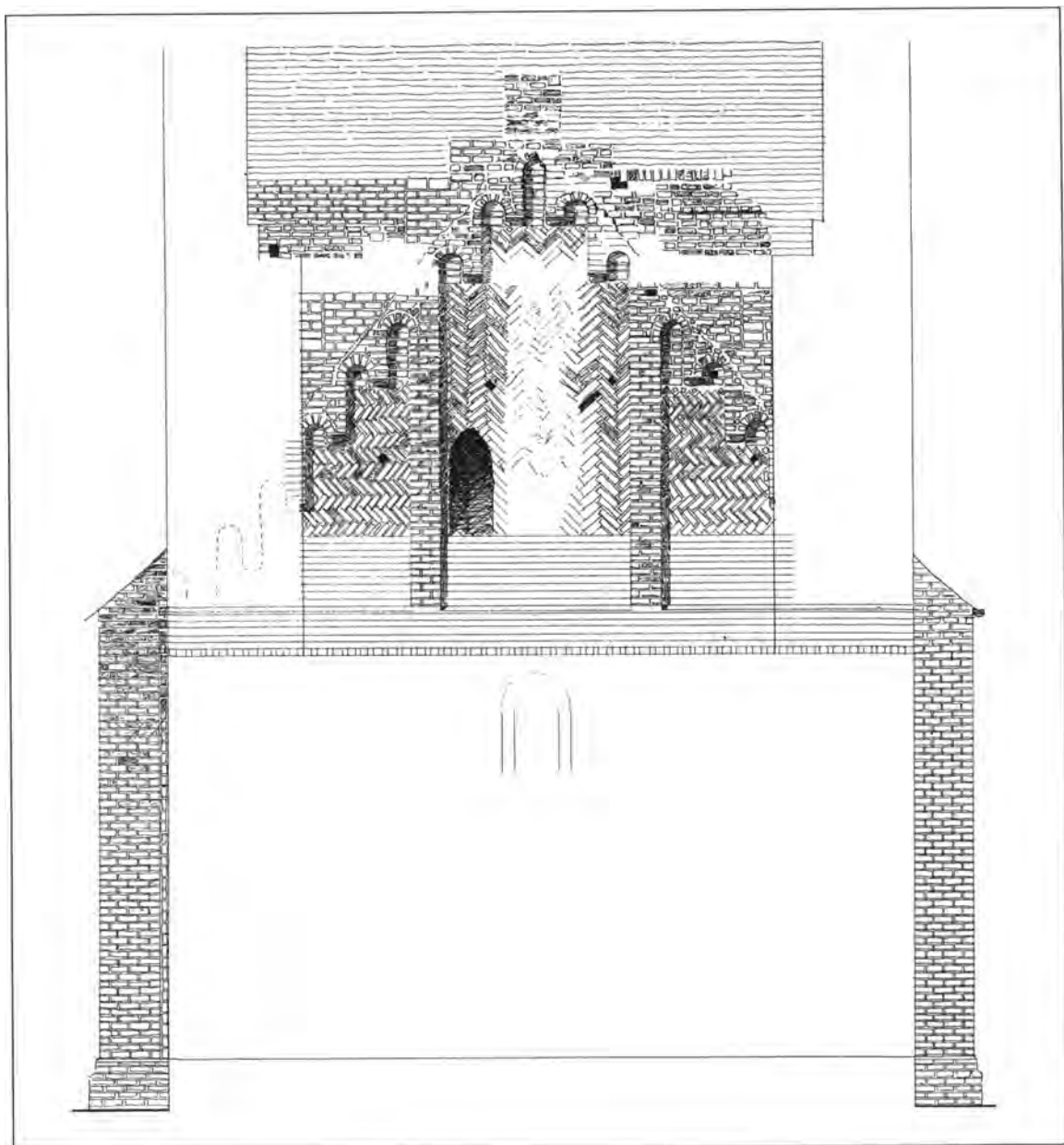
Fig. 10. Skibets vestgavl før restaurering (s. 3352). 1:100. Opmåling ved A. Clemmensen o. 1880. Se også fig. 75. - The nave's west gable before restoration.
