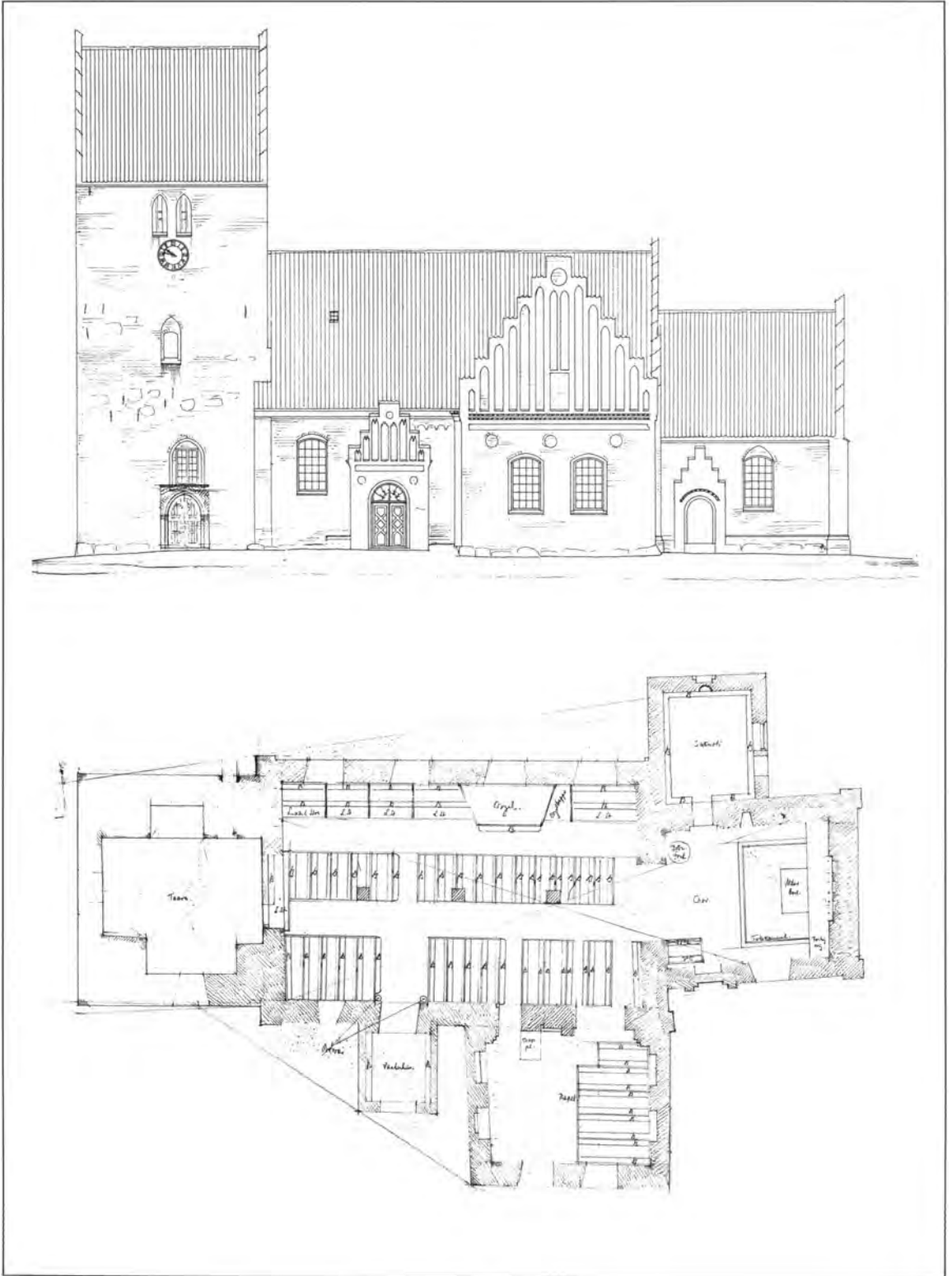
Fig. 21a-c. Opmålinger af kirken før restaureringen 1:300. Plan, sydfacade og nordfacade. A. Clemmensen o. 1879. - a-c. Measured drawings of the fabric prior to the restoration. Ground-plan, south facade and north facade. 1879.
