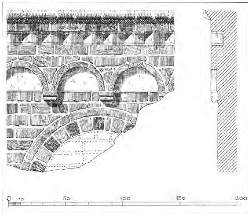
Fig. 8. Skibets buefrise og et vinduesstik, set fra kapellets loft. 1:20 Tegning af C. G. Schultz 1929. - Blind arcade in the nave and voussoirs of a window seen from the loft above the chapel.
