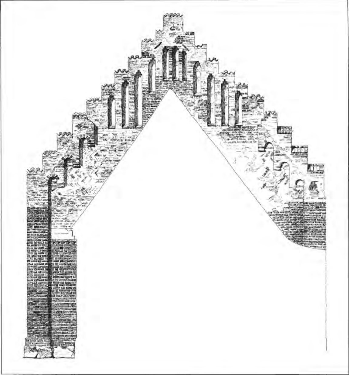
Fig. 7. Skibets østgavl før restaurering (s. 3352). 1:100. Opmåling ved A. Clemmensen o. 1880. - The nave's east gable before restoration.
