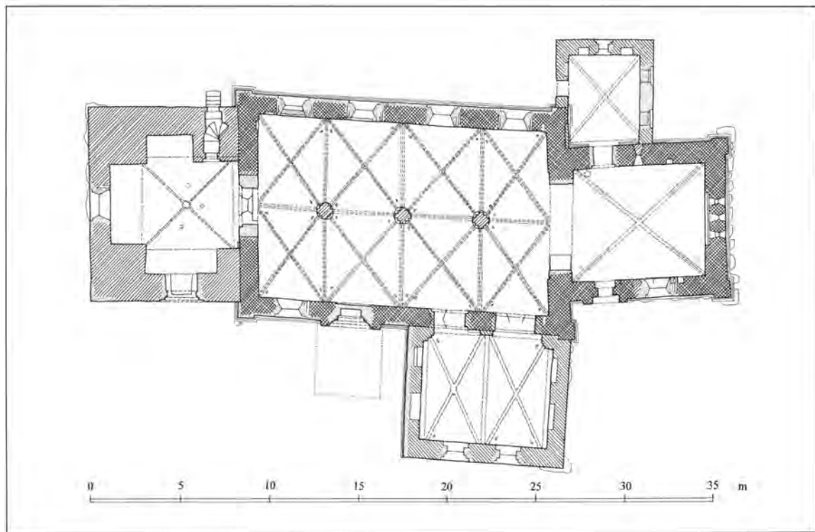
Fig. 5. Plan 1:300. Målt af C. G. Schultz 1929. Suppleret og tegnet af Peter Kristiansen 1995. Signaturforklaring s. 9. - Ground-plan. Key on p. 9.
