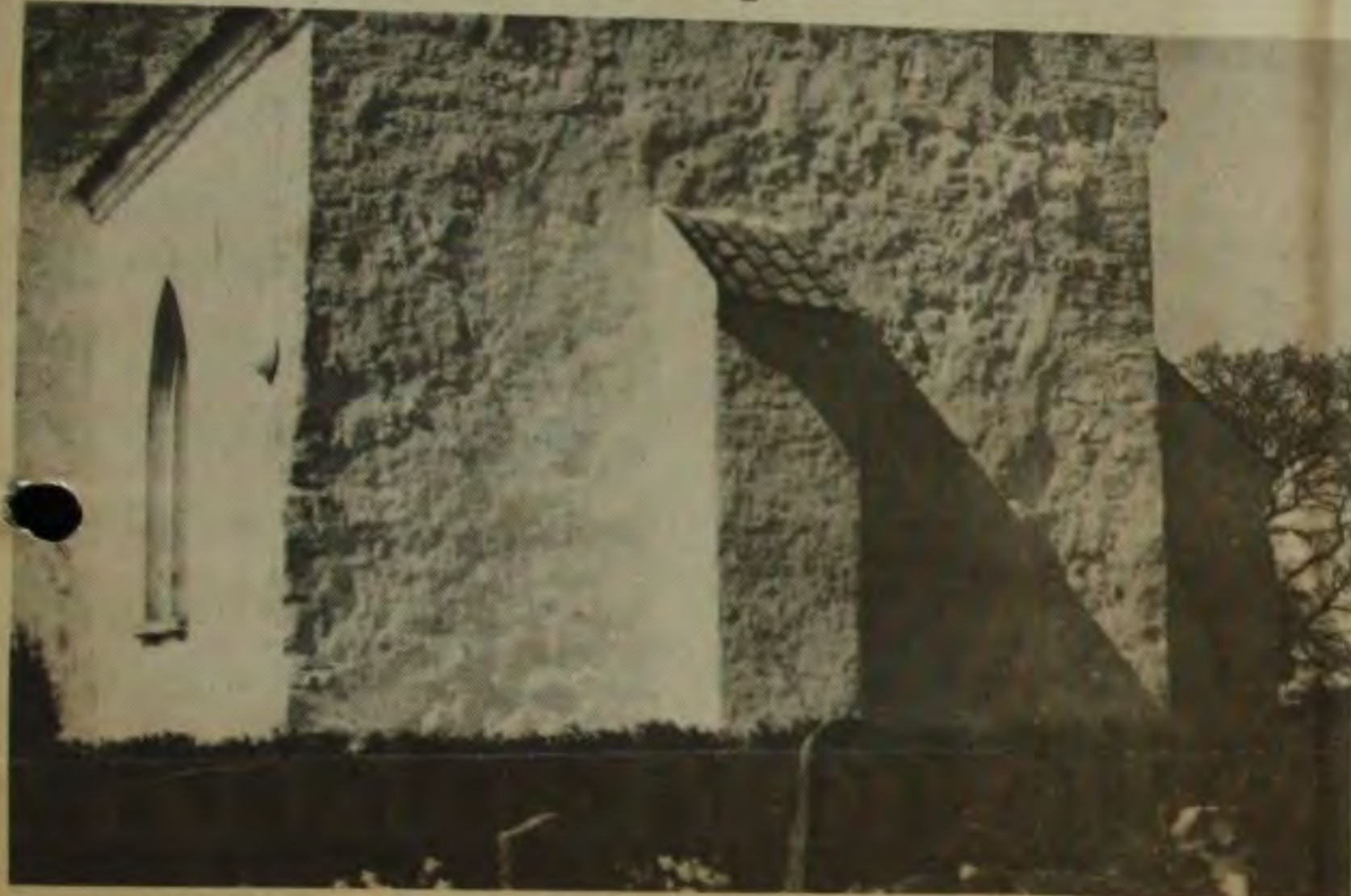
En stræbepille holder på Nr. Asmindrup kirkes kampestensmur.
